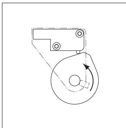
6-12.5 Kierunek sterowania krzywki sterującej S1 - wyłącznik krańcowy bezpieczeństwa brama-otwarta
