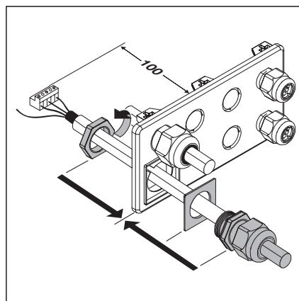
4-2.6 Montaż końcowy do pokrywy obudowy sterowania
