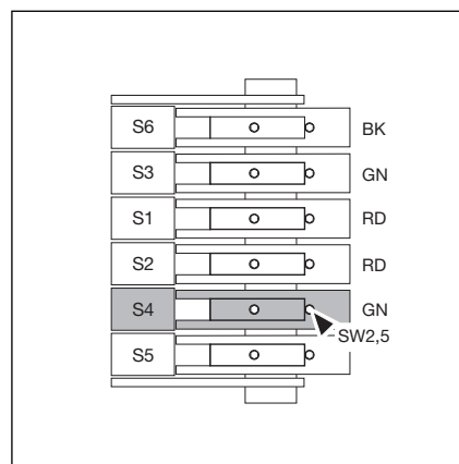
6-16.1 Ustawienie dokładne wyłącznika krzywkowego S3 -Polozenie krancowe Brama zamknieta-
