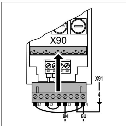
4-6.5 Typ silnika S25WS: Podłączenie jednofazowego prądu przemennego do X90
