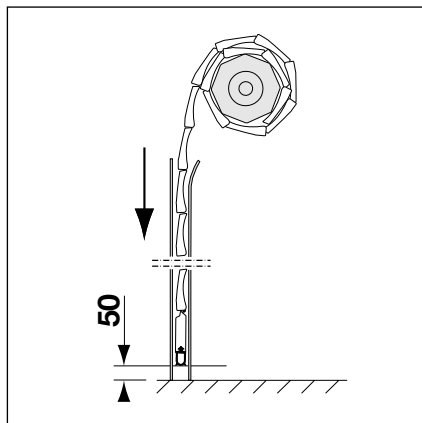
6-14.2 Pozycja SKS-Stop
