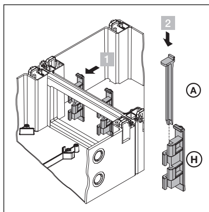
3-3.2 Montaż
