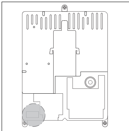
4-3.2 Położenie podłączenia silnika wewnątrz obudowy sterowania
