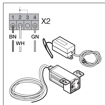
4-5.3 Podłączenie odbiornika sygnałów radiowych
