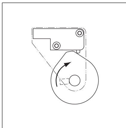
6-14.3 Kierunek sterowania krzywki sterującej S6 - SKS-Stop -
