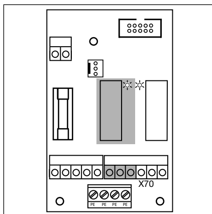
6-24.1 Przełącznik 1 płyty wielofunkcyjnej
