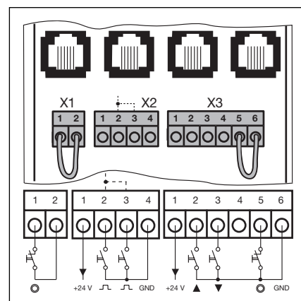
4-5.2 Podłączenie zacisków śrubowych
