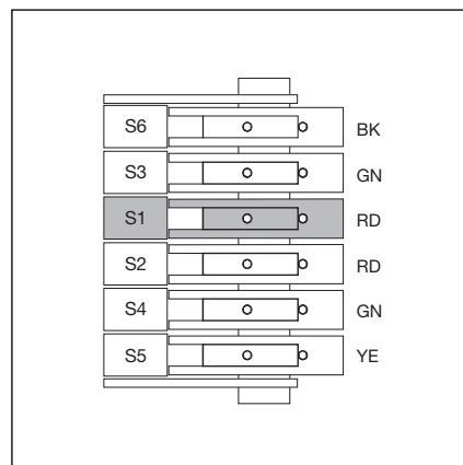
6-12.4 Krzywka sterująca S1 - wyłącznik krańcowy bezpieczeństwa brama-otwarta -
