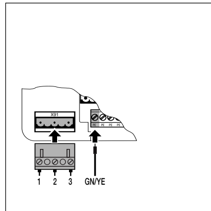
4-3.3 Podłączenie przewodu silnika do X91
