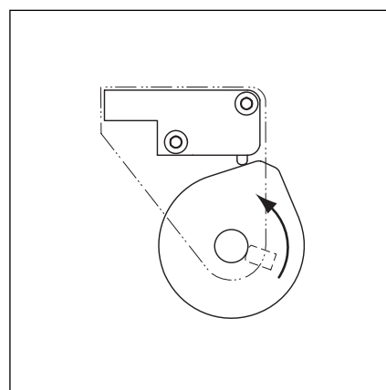
6-12.2 Kierunek sterowania krzywki sterującej S3 - położenie krańcowe brama-otwarta -
