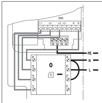
4-6.9 Typ silnika K09WS: należy dokonać przebiegunowania podłączenia sieci prądu zmiennego 1-fazowego do wyłącznika głównego!
