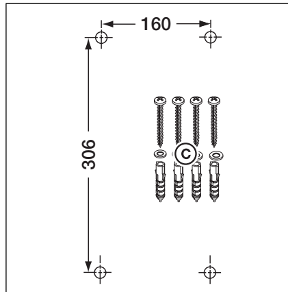
3-2.6 Obraz nawiercanych otworów montażowych, potrzebne elementy montażowe
