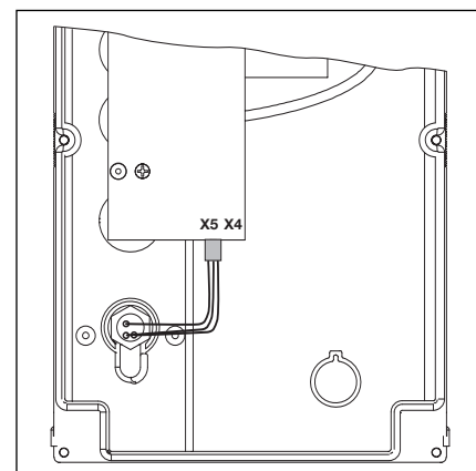
5-1.3 Podłączenie włącznika na klucz do X5 na płytce obwodu elektronicznego klawiatury
