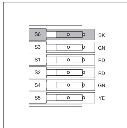
6-14.2 Krzywka sterująca S6 - SKS-Stop -
