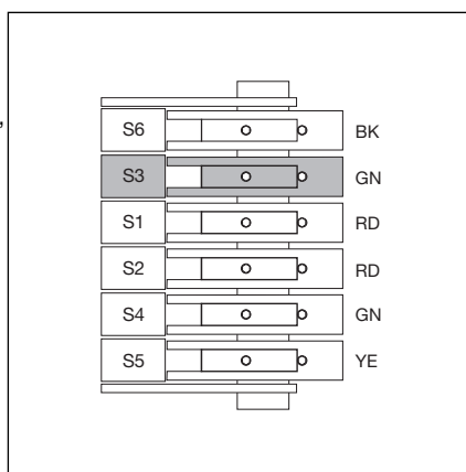
6-12.1 Krzywka sterująca S3 - położenie krańcowe brama-otwarta -
