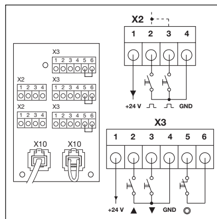
4-4.2 Podłączenie dodatkowych zewnętrznych elementów obsługi do X10
