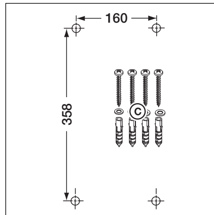
3-1.6 Obraz nawiercanych otworów montażowych, potrzebne elementy montażowe
