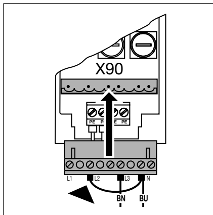
4-6.6 Typ silnika K09WS: należy dokonać przebiegunowania podłączenia sieci prądu zmiennego 1-fazowego do X90!
