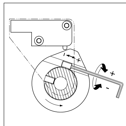
6-15.3 Ustawienie dokładne wyłącznika krzywkowego S3 -krańcowe Brama otwarta-
