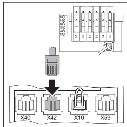
4-3.7 Podłączenie przewodu systemowego wyłącznika krańcowego krzywkowego do X42
