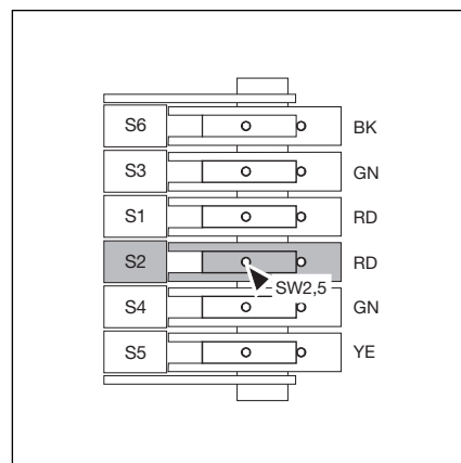
6-13.6 Unieruchomić krzywkę
