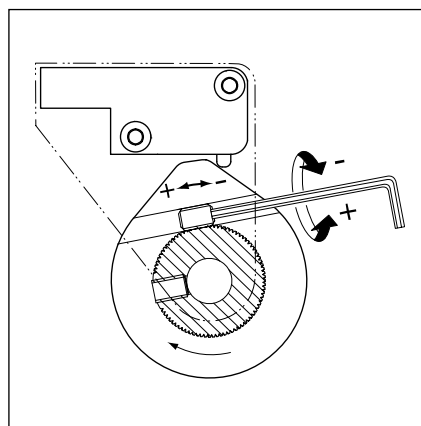
6-16.3 Ustawienie dokładne wyłącznika krzywkowego S3 -Polozenie krancowe Brama zamknieta-
