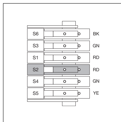
6-13.4 Krzywka sterująca S2 - wyłącznik krańcowy bezpieczeństwa brama-zamknięta -
