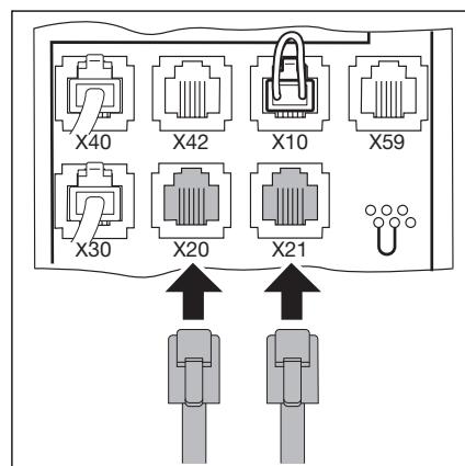
4-4.3 Podłączenie urządzeń zabezpieczających przy pomocy styków systemowych
