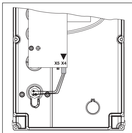
6-23.1 Podłączenie miniaturowego zamka, strona wewnętrzna pokrywki, przełożyć wtyki z X5 do X4.
