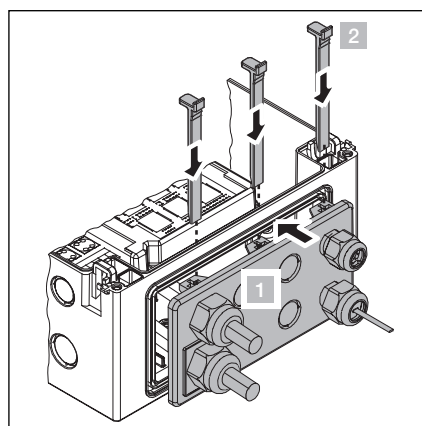
4-2.9 Zamontować pokrywę obudowy
