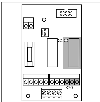
6-25.1 Przekaźnik 2 płytki wielofunkcyjnej
