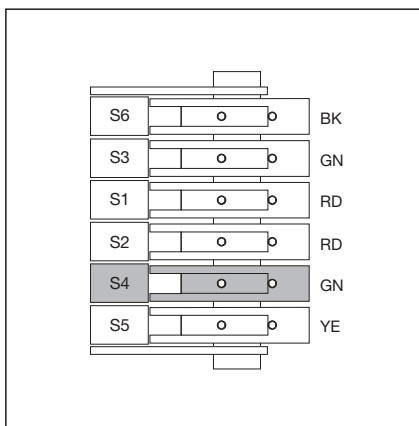
6-13.1 Krzywka sterująca S4 - położenie krańcowe brama-zamknięta -
