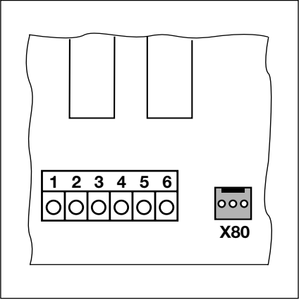
7-4.2 Podłączenie do istniejących płytek poprzez X80
