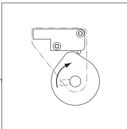
6-13.5 Kierunek sterowania krzywki sterującej S2 - wyłącznik krańcowy bezpieczeństwa brama-zamknięta
