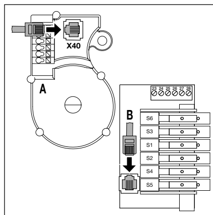
4-2.3 4-2.3 Podłączenie przewodu systemowego do gniazda przyłączeniowego - A = czujnika pozycji bramy - B = wyłącznika krańcowego krzywkowego
