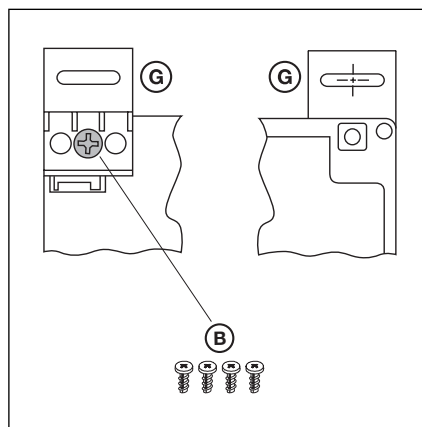
3-1.5 Mocowanie podór montażowych, widok z tyłu, widok z przodu
