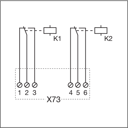
7-4.3 Schemat połączeń przełączników
