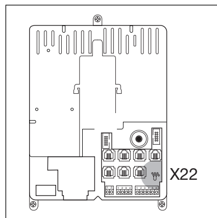
5-3.1 Usytuowanie mostka z drutu X22
