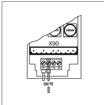
4-6.3 Podłączenie żył przewodu uziemiającego w przewodzie sieciowym
